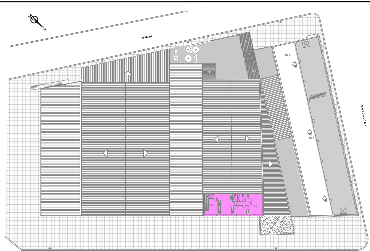
PLANTA SEGONA
