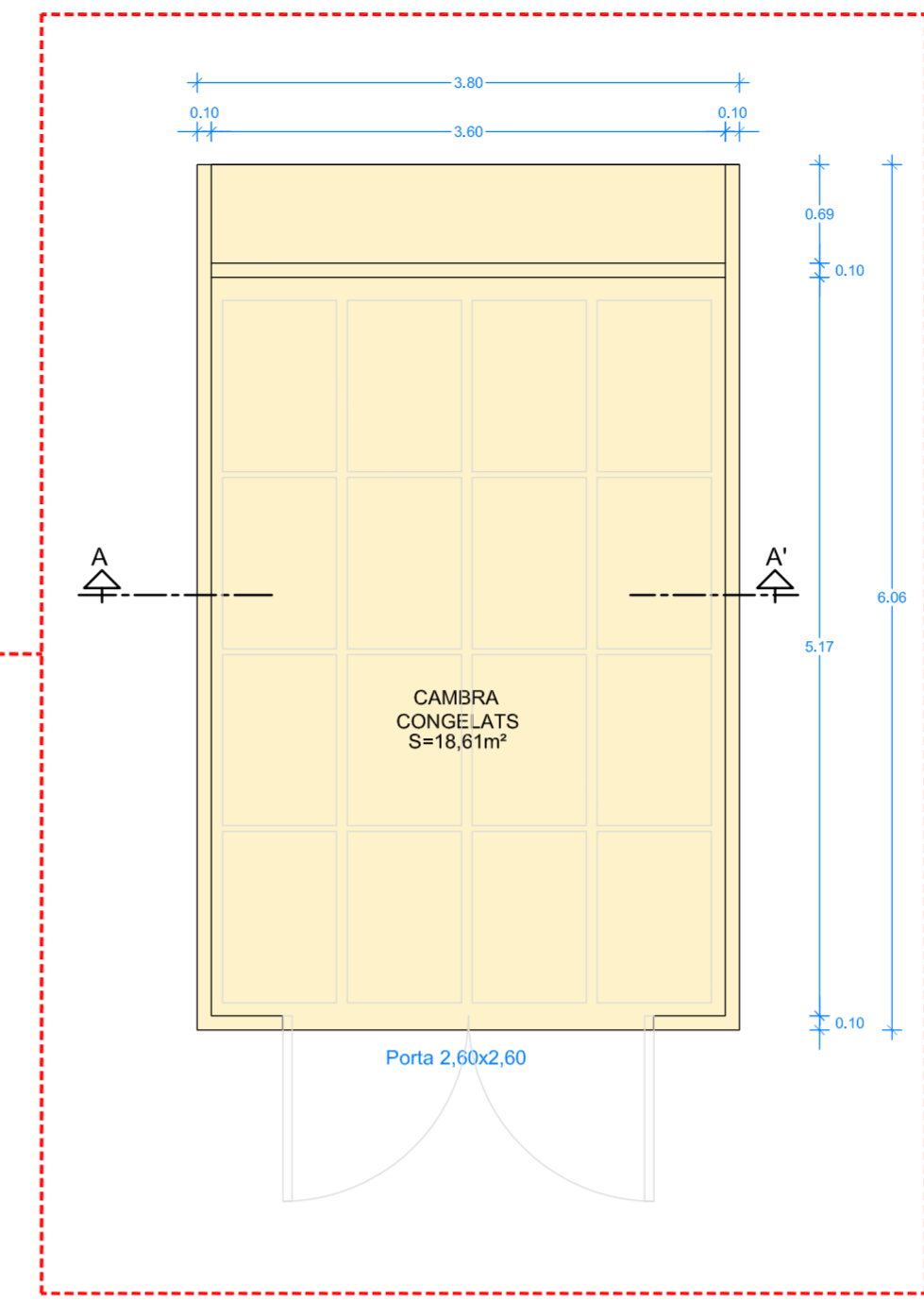
DETALL ÀMBIT D'ACTUACIÓ E: 1/50
