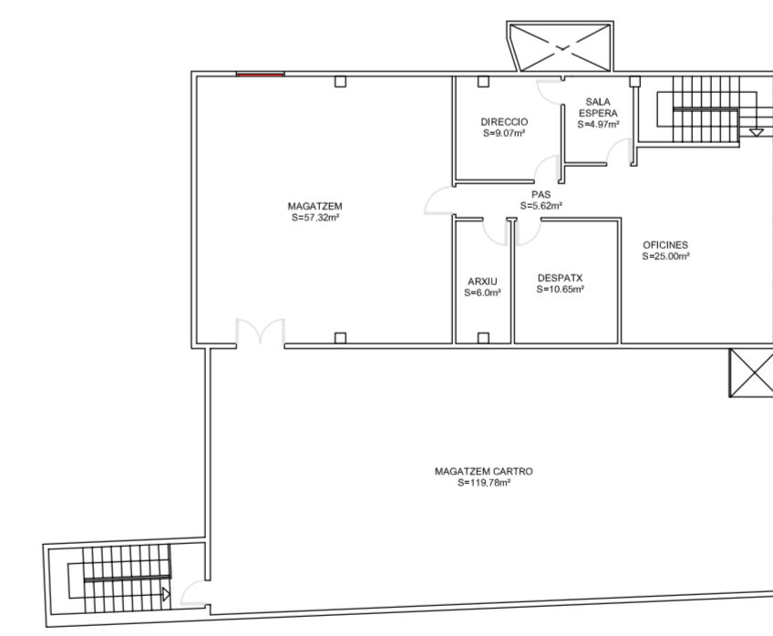
PLANTA ALTELL E: 1/200
