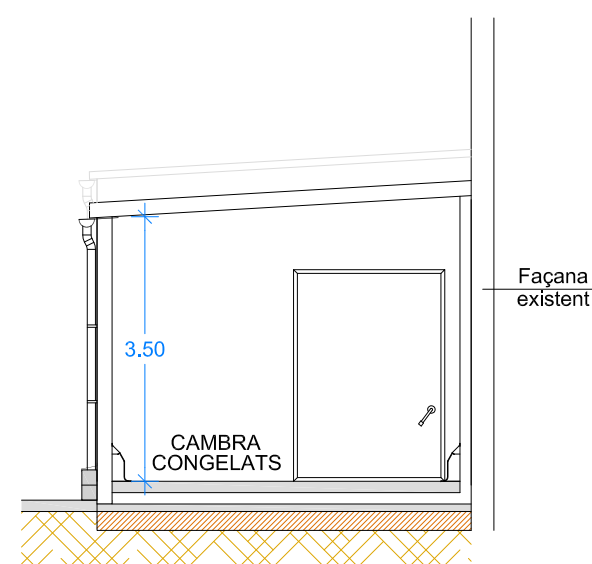
SECCIÓ A-A' E: 1/100
