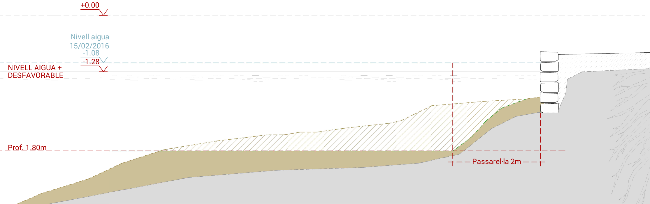
SECCIÓ PER PART NO ESFONDRAADA
