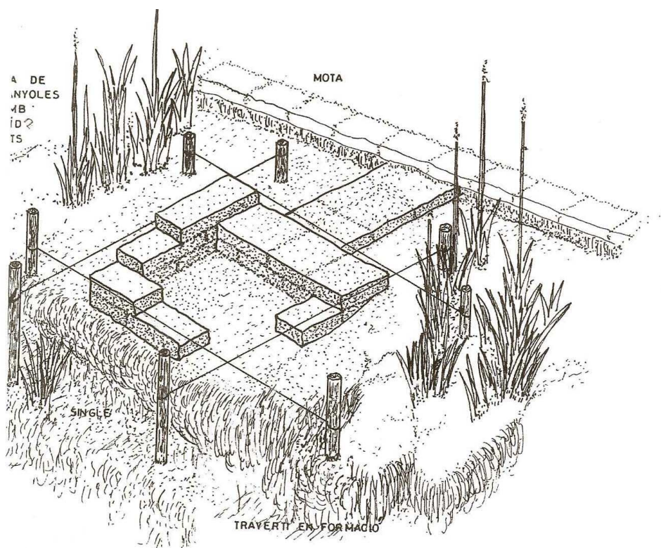
Construcció d'una pesquera en zona de travertins en formació
