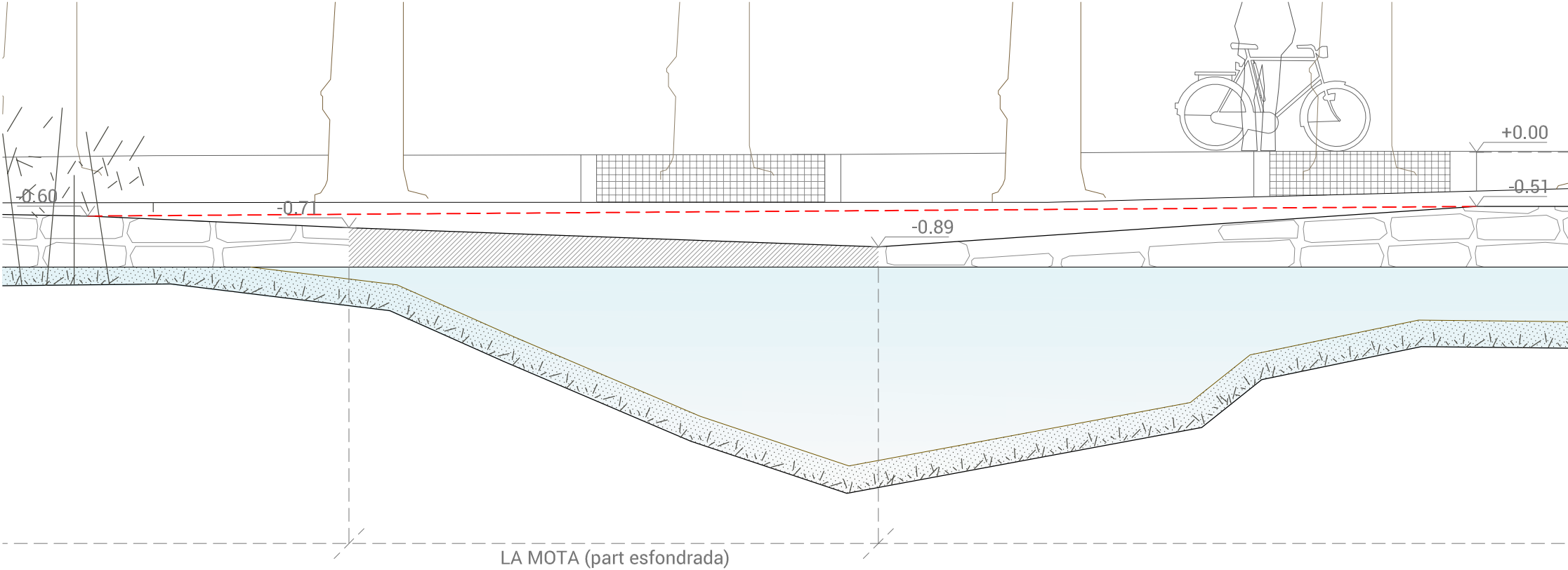
SECCIÓ 1 LONG.
