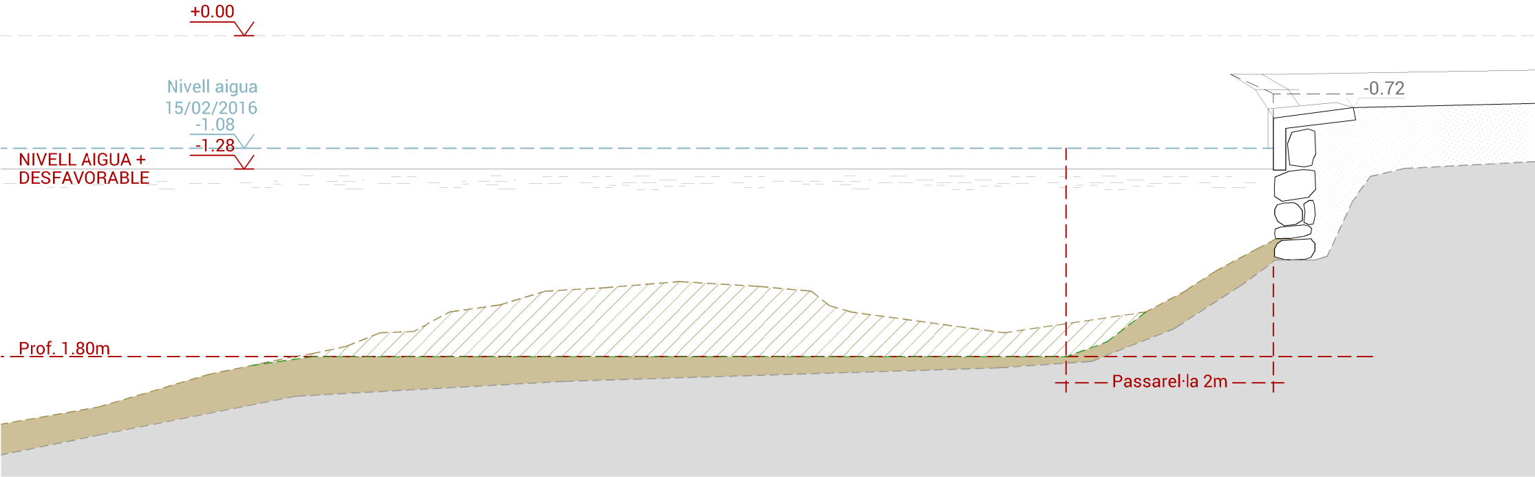
SECCIÓ PER PART ESFONDRAADA
