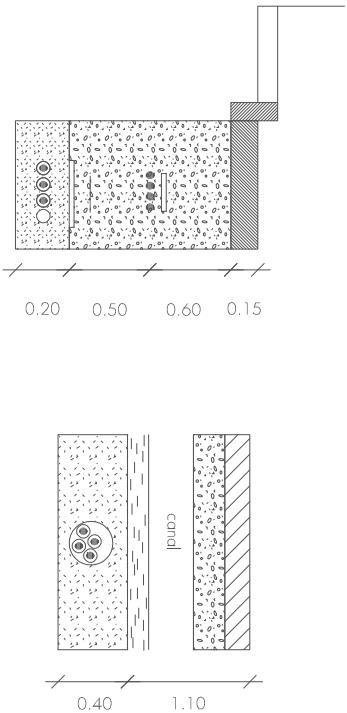
DETALL LÍNIA SUBTERRÀNIA A 25kV
