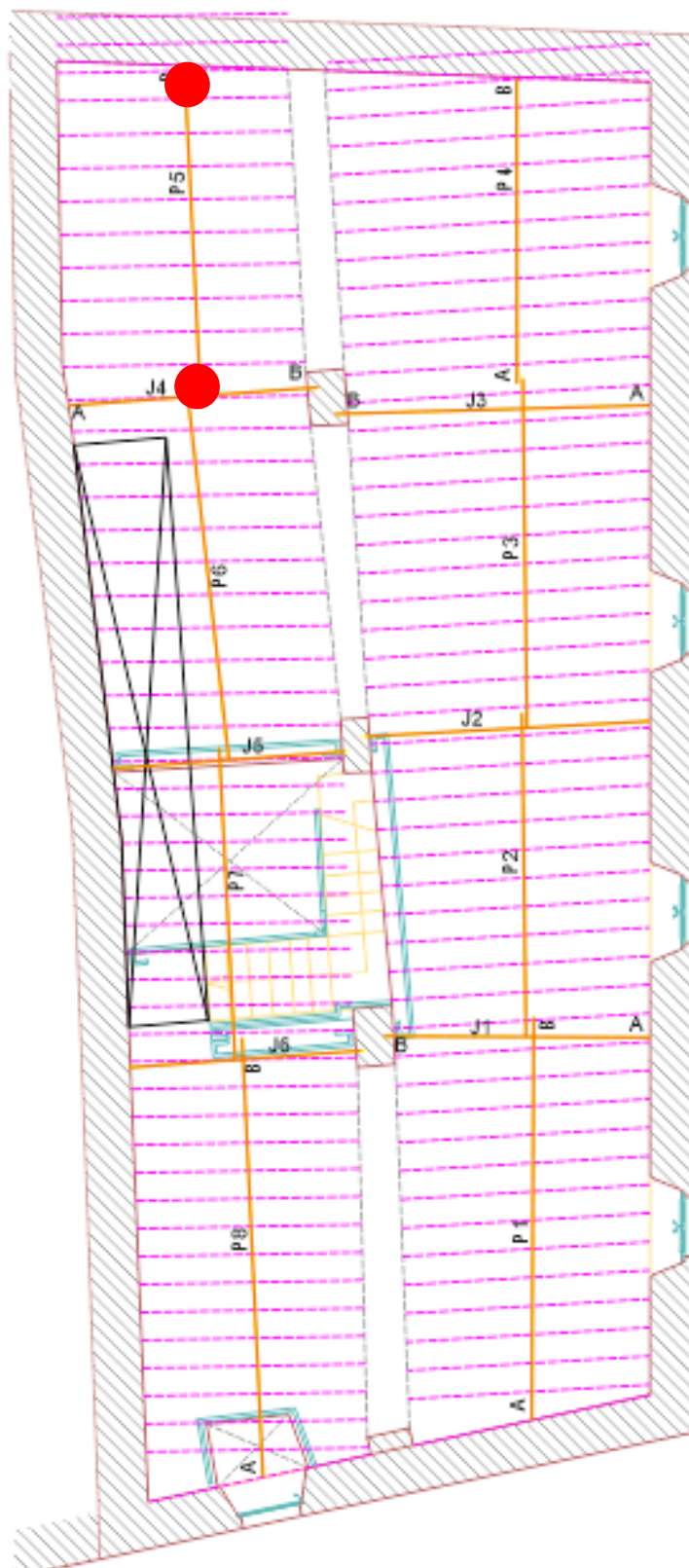
Croquis de disfuncions d'elements. Jàsseres i Partillums
