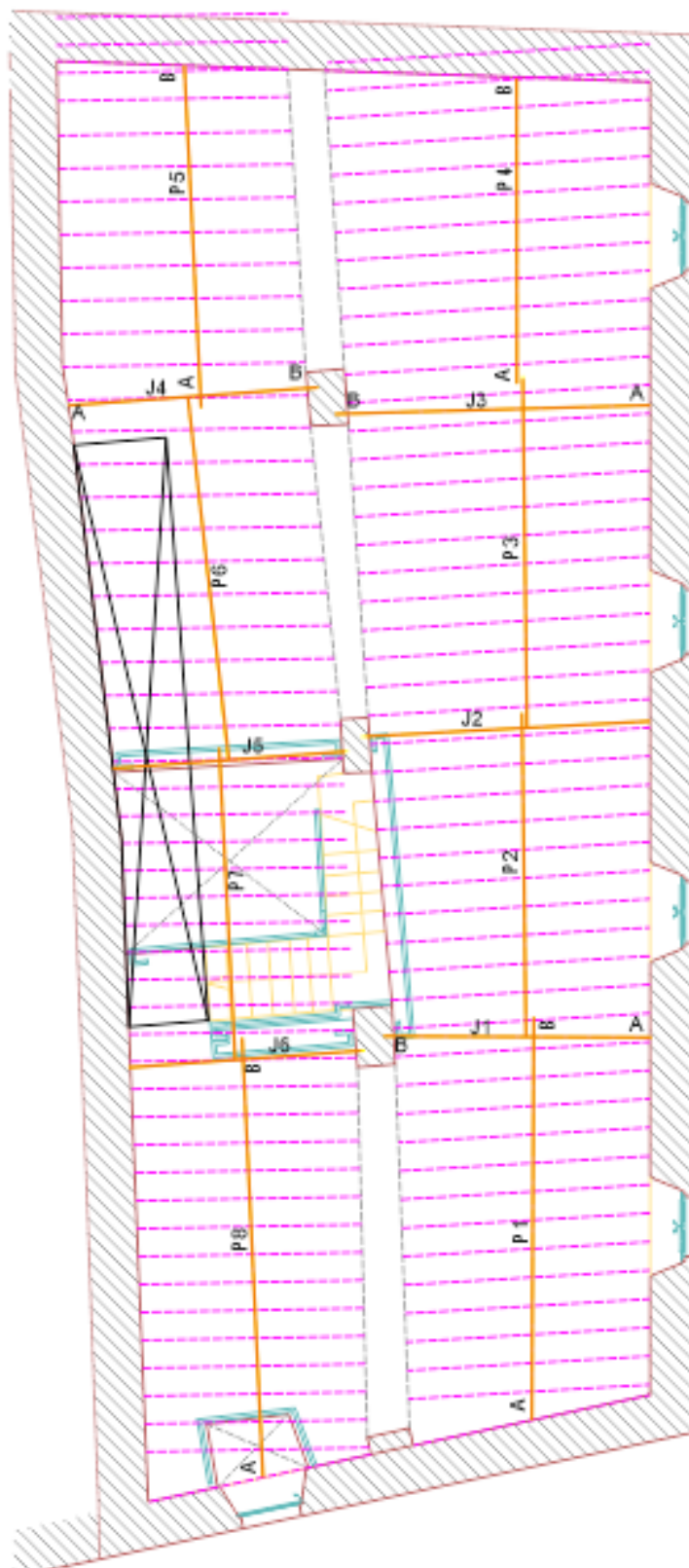
Croquis de situació d'elements. Jasseres i Partills
