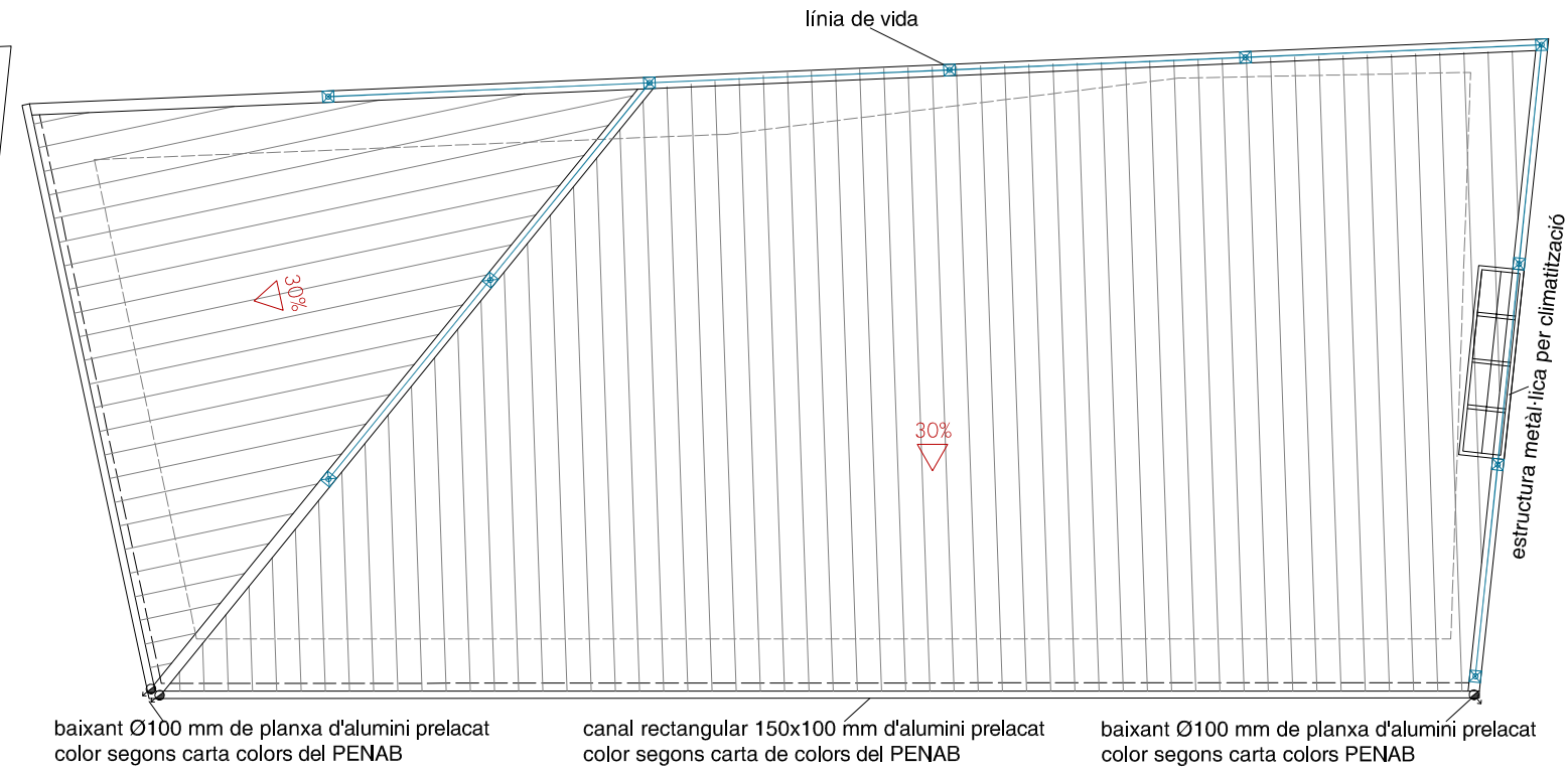
PLANTA COBERTA PROPOSADA
