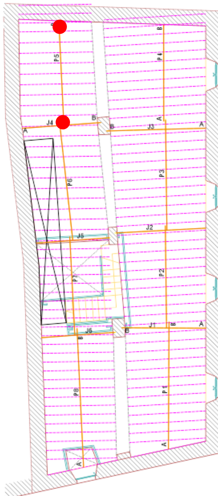
Croquis de disfuncions d'elements. Jàsseres i Partillums
