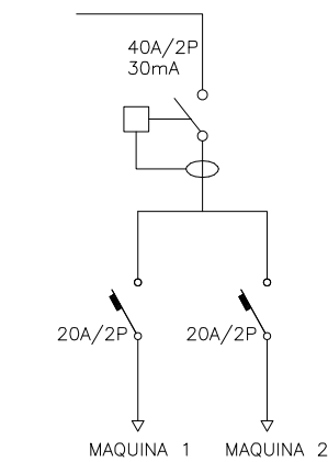
ESQUEMA ELÈCTRIC
