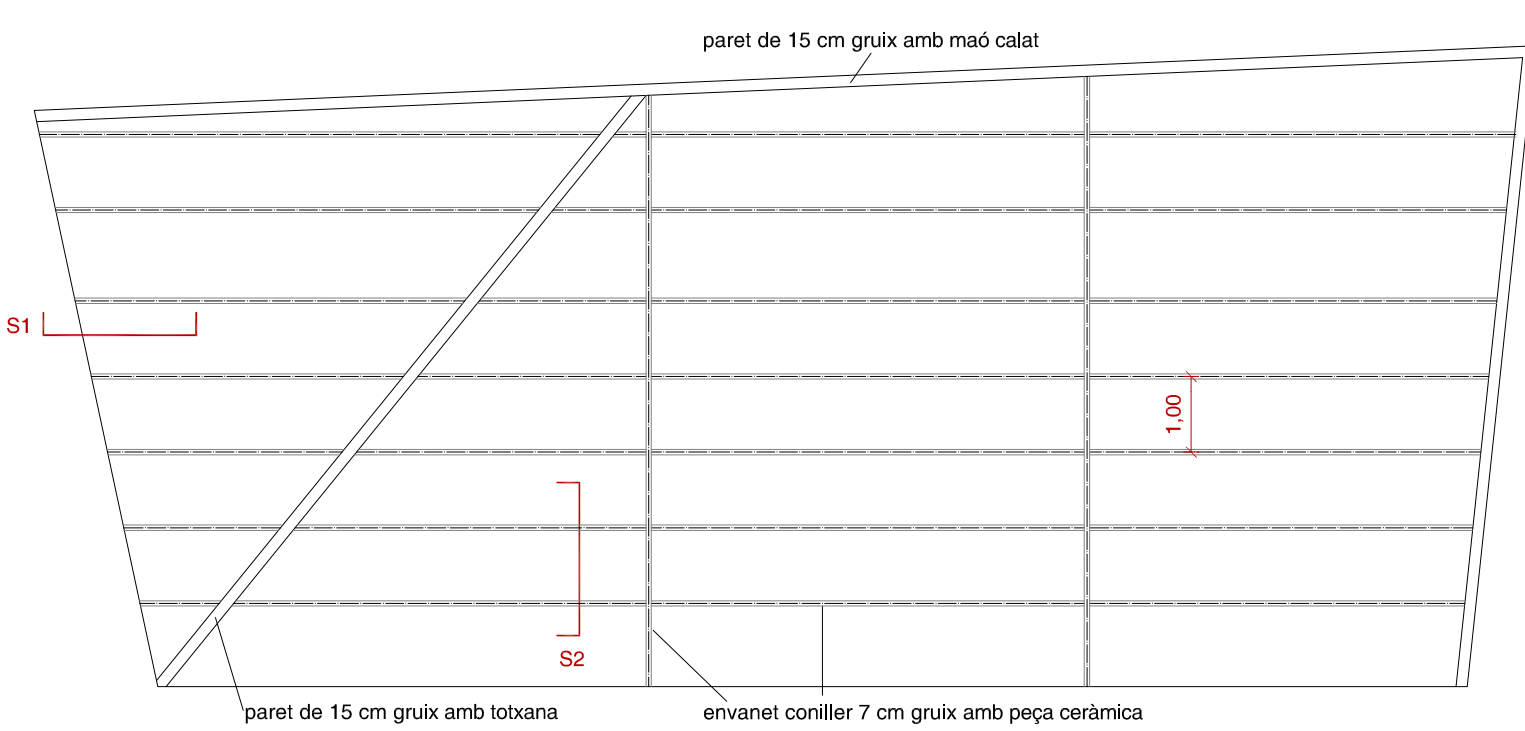
PLANTA ENVANETS CONILLERS
