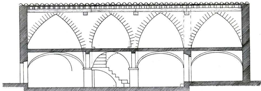
SECCIÓ LONGITUDINAL
