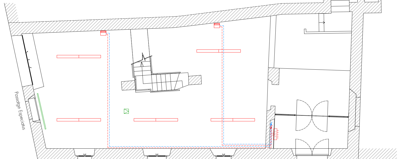
PLANTA BAIXA
